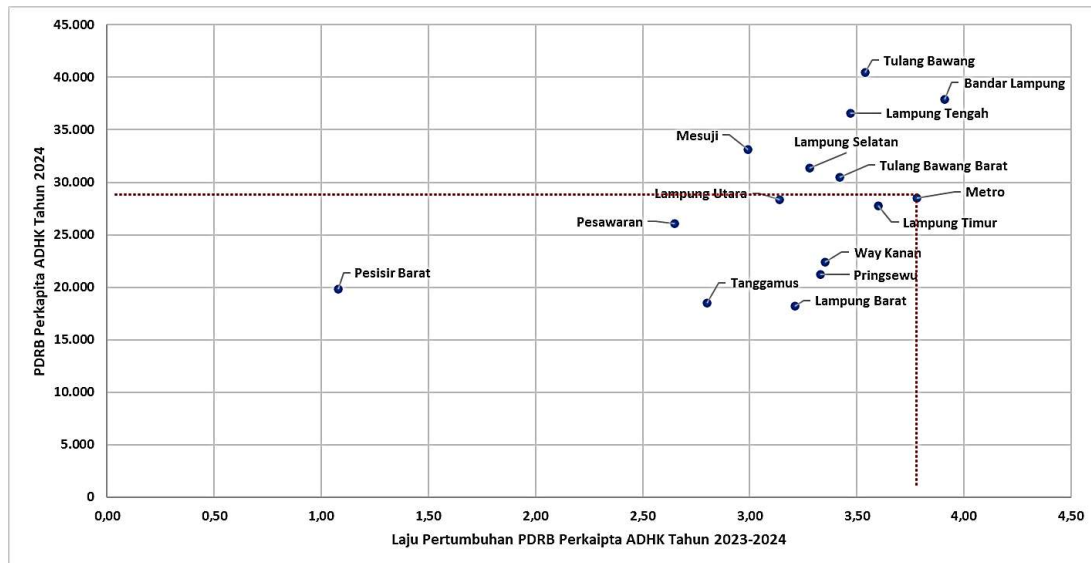
Grafik 2.6 Perbandingan PDRB per kapita ADHB dengan Laju Pertumbuhan PDRB per kapita ADHB Kabupaten/Kota se Provinsi Lampung Tahun 2023-2024
