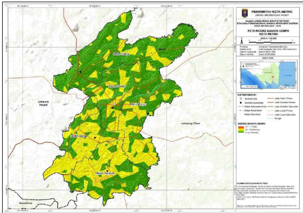
Gambar 2.12 Peta Indeks Bahaya Gempa Kota Metro
