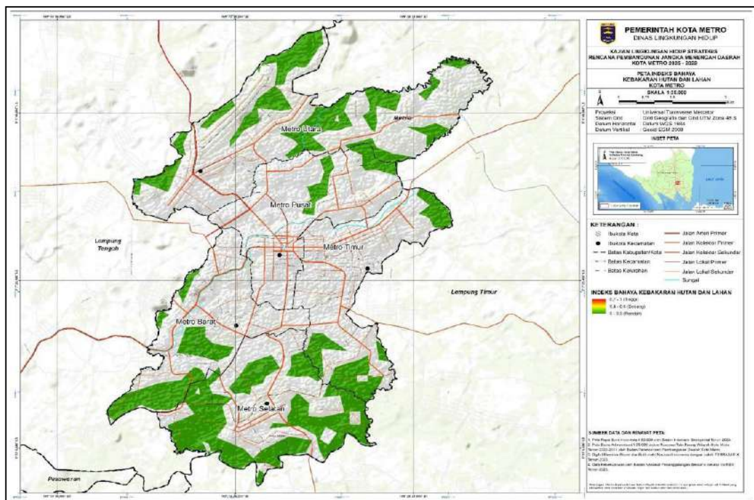
Gambar 2.10 Peta Indeks Bahaya Kebakaran Hutan dan Lahan Kota Metro
