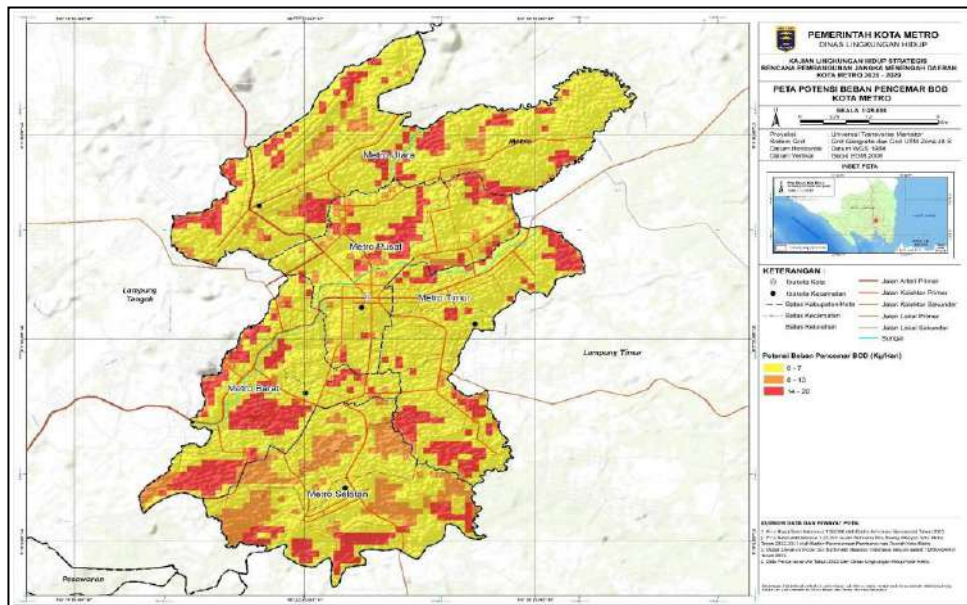
Gambar 2.14 Potensi Beban Pencemar Zat BOD Kota Metro
