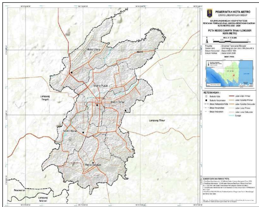
Gambar 2.11 Peta Indeks Bahaya Longsor Kota Metro
